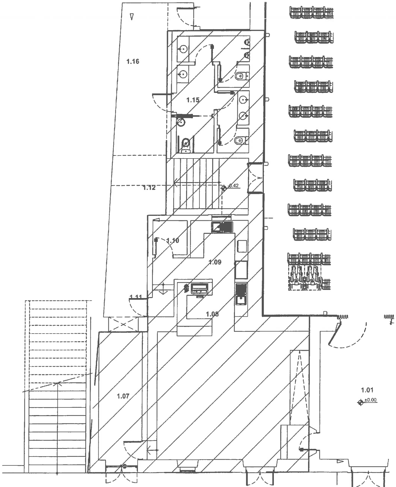
PLANTA DO PISO 1
